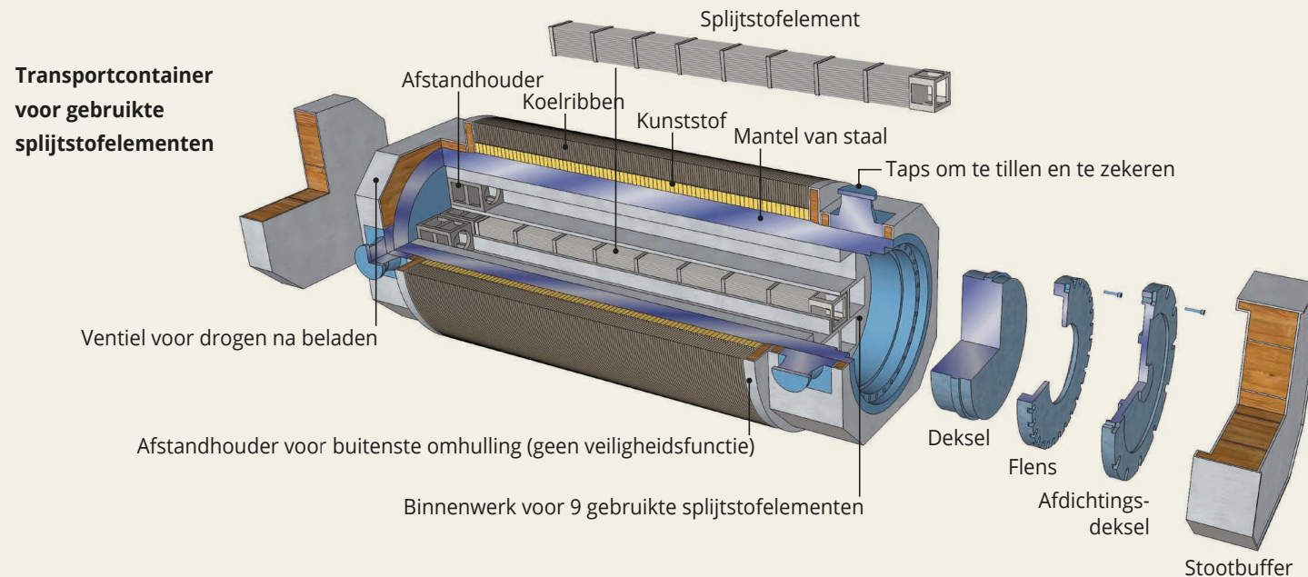
Figuur 6.2. Container van EPZ voor het vervoeren van gebruikte splijstofelementen (Bron: EPZ).
