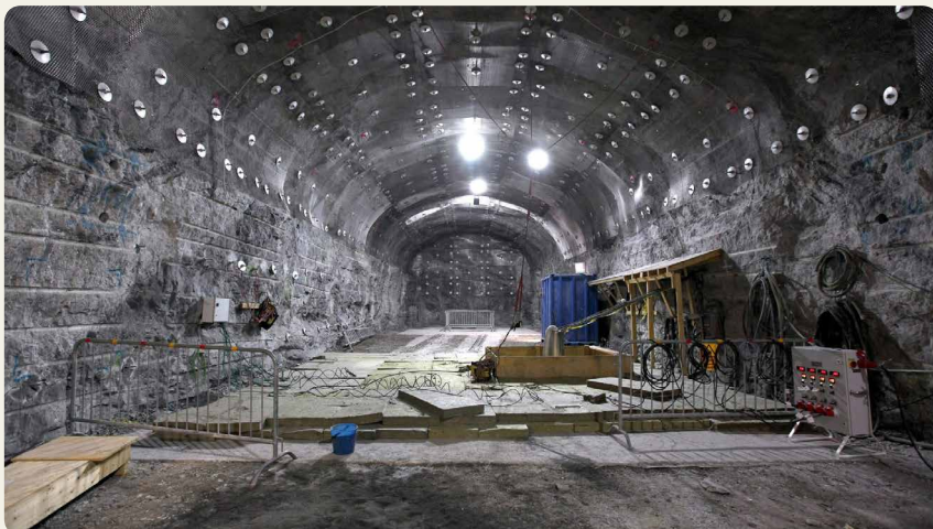
Ondergrondse eindberging in aanbouw (Finland)
